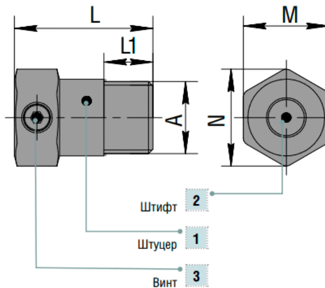
Габаритные размеры устройства дренажного серии УС
