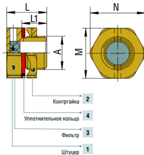
Габаритные размеры устройства дренажного серии УСЕ
